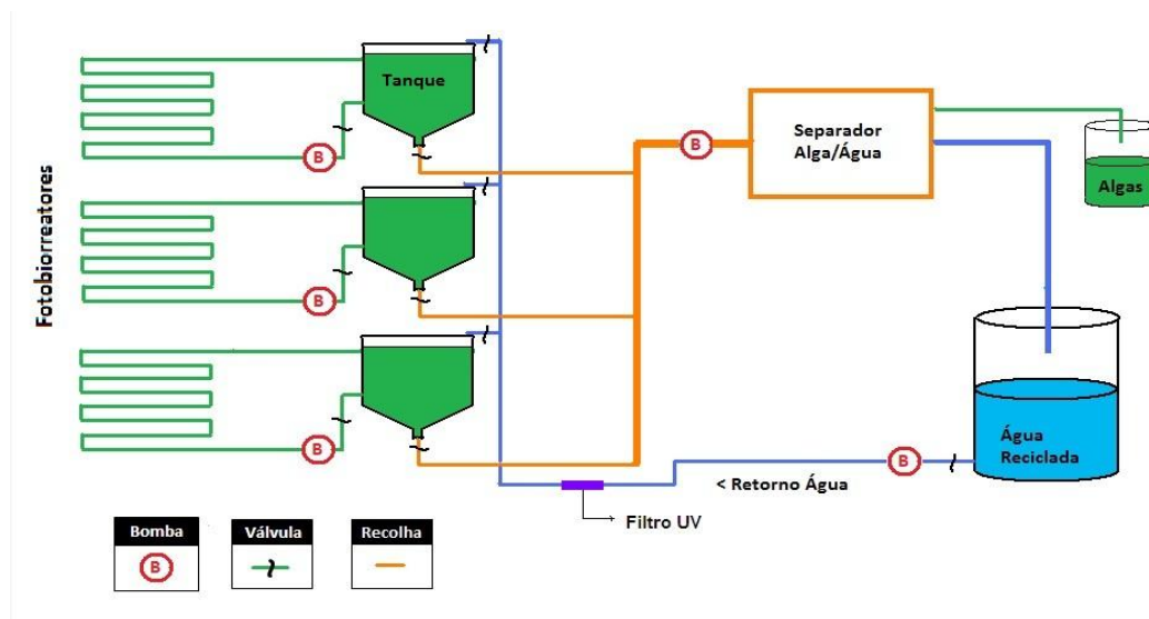
Figura 03: Esquema dos fotobiorreatores e reciclagem de água
